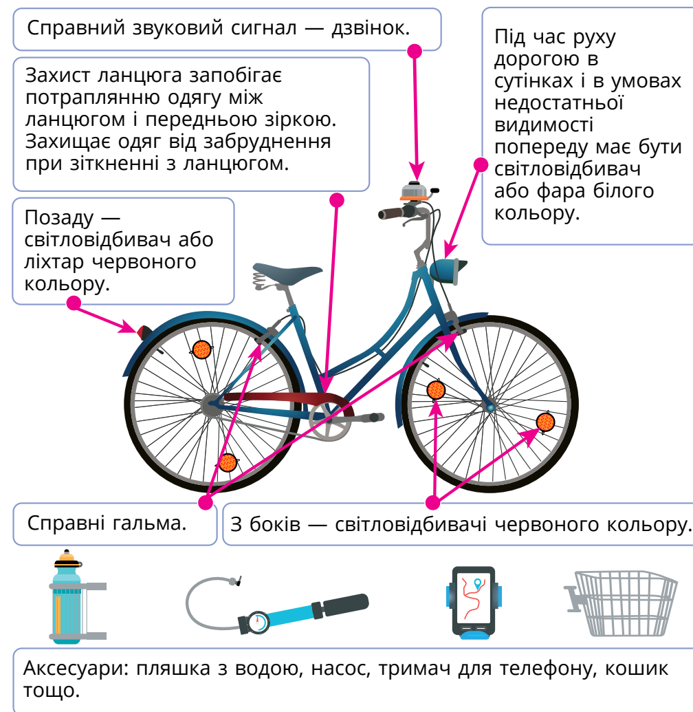
Мал. 94. Оснащення велосипеда
