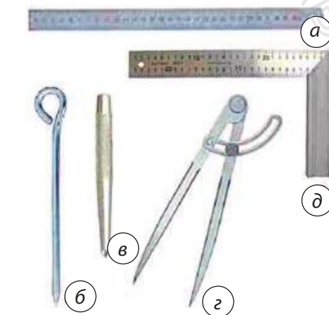
Мал. 15.2. Інструменти, необхідні для розмічання жерстяної поверхні: а — лінійка; б — рисувальні; в — кернер; г — циркуль; д — кутник
